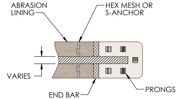
EDGE-TAB
