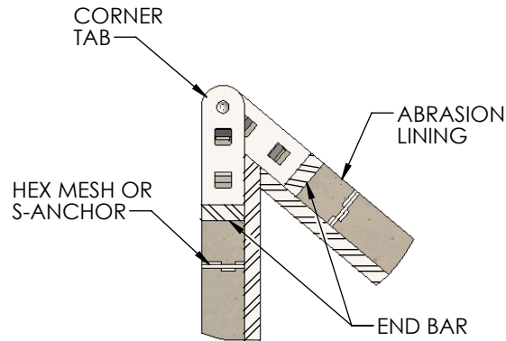
CORNER EDGE
